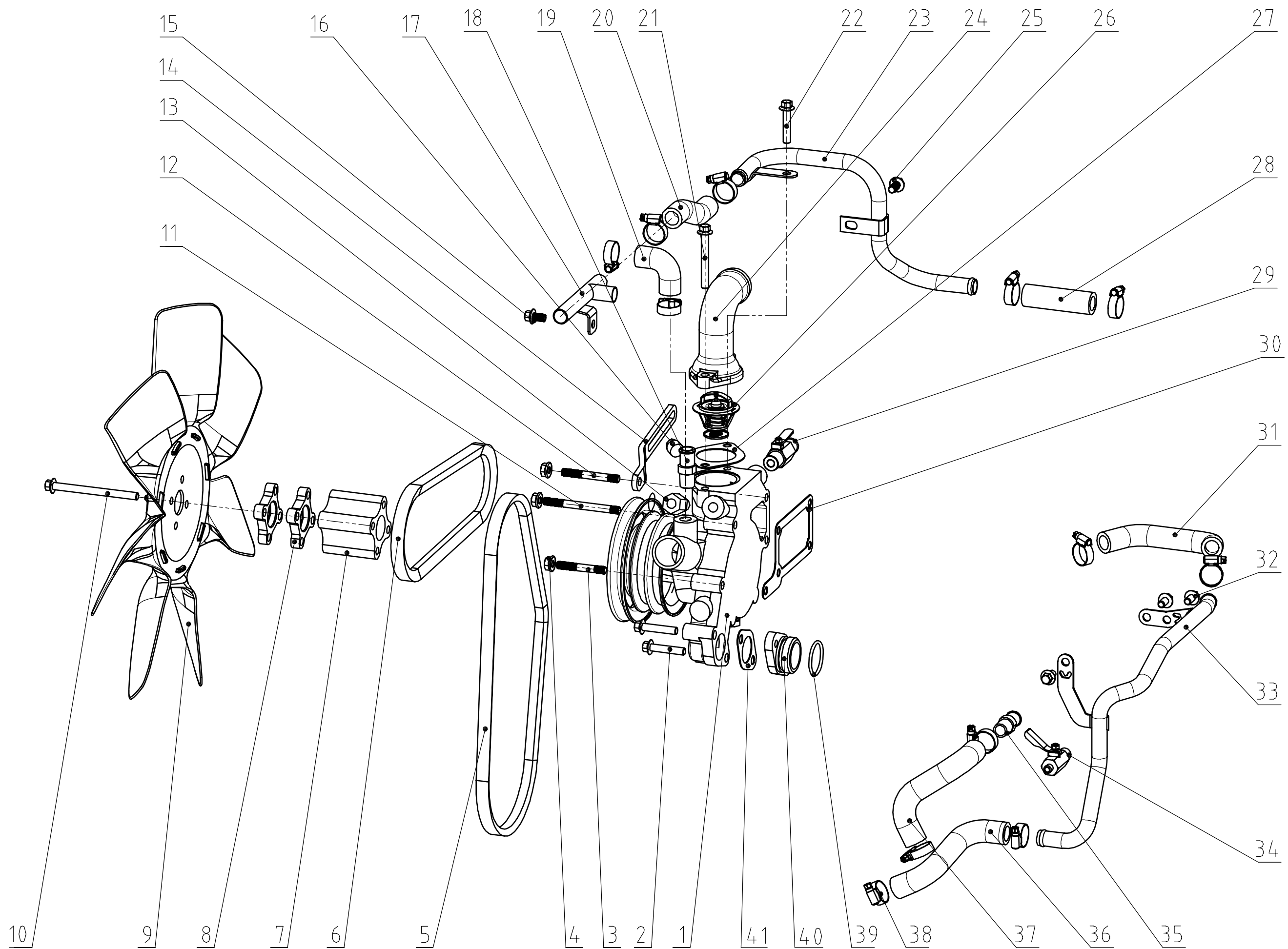
4L28V50-06000 冷却系统总成
