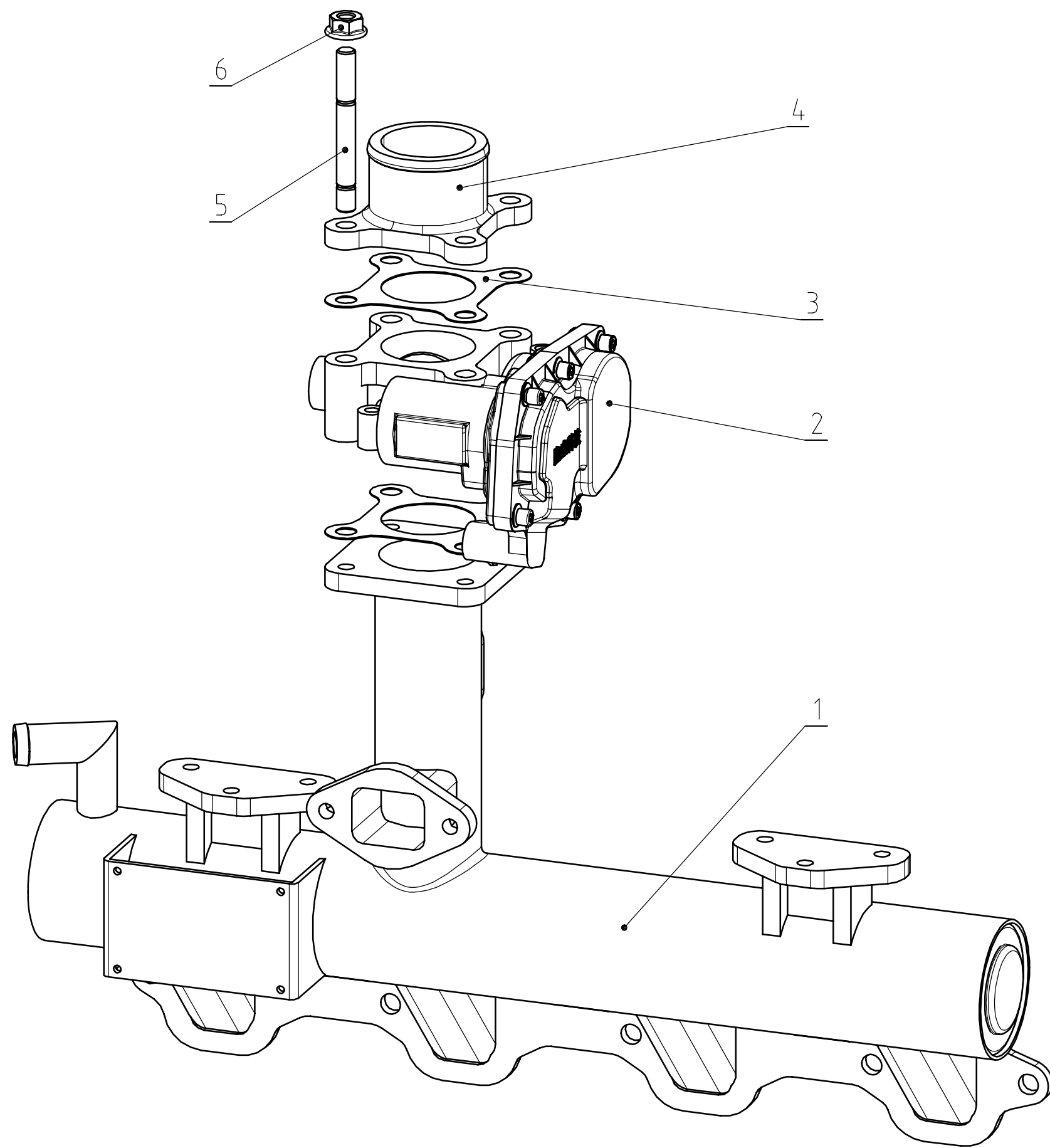
4L28V50-07000 进气系统总成
